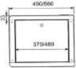
Yan görünüş
